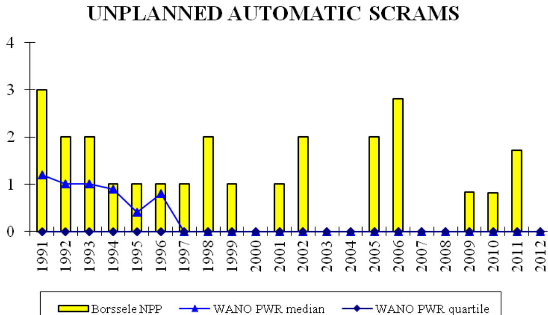
Figuur 1 Noodstops kerncentrale Borssele als voorbeeld storingen
