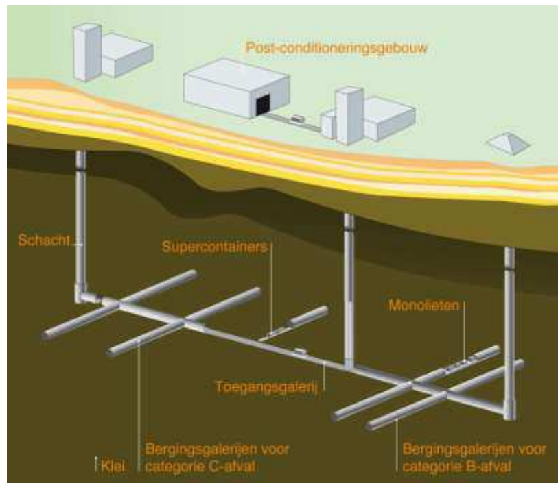
Schematische schets mogelijke eindberging België
