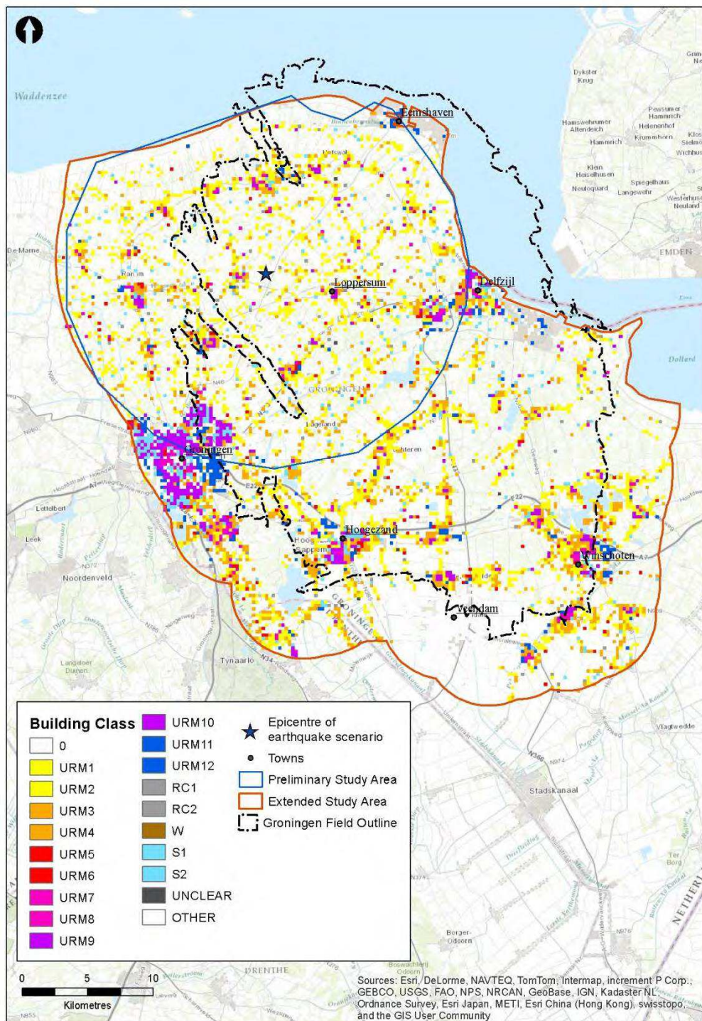
Figuur 2: Ruimtelijke verdeling van de verschillende typen huizen in de studie gebieden van ARUP (figuur A.3 [6]). De 12 verschillende niet-versterkte bakstenen huizen (URM) kunnen op basis van bouwperiode worden onderverdeeld in 3 kwetsbaarheidsgroepen: gebouwd voor 1920, gebouwd tussen 1920 en 1960 en gebouwd na 1960. 90% van de bebouwing binnen een straal van 15 km van het epicentrum van de Huizinge beving en 77% van de bebouwing in het gebied tot 5 km van de rand van het Groningen gasveld vallen binnen deze URM categorie. Deze categorie huizen is het meest gevoelig voor schade ten gevolge van aardbevingen.
